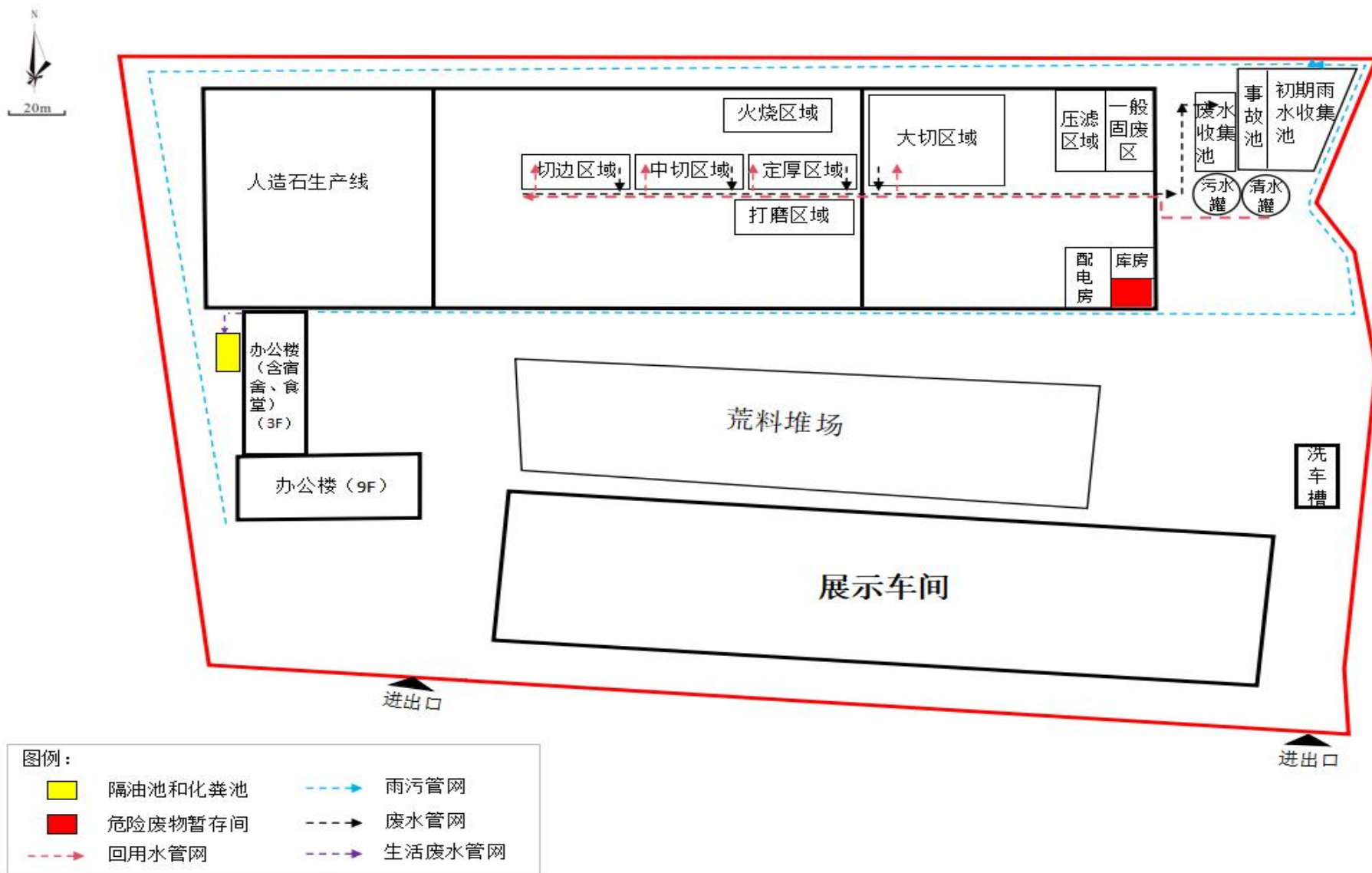
附图 3 项目总平面布置图及雨污管网图
