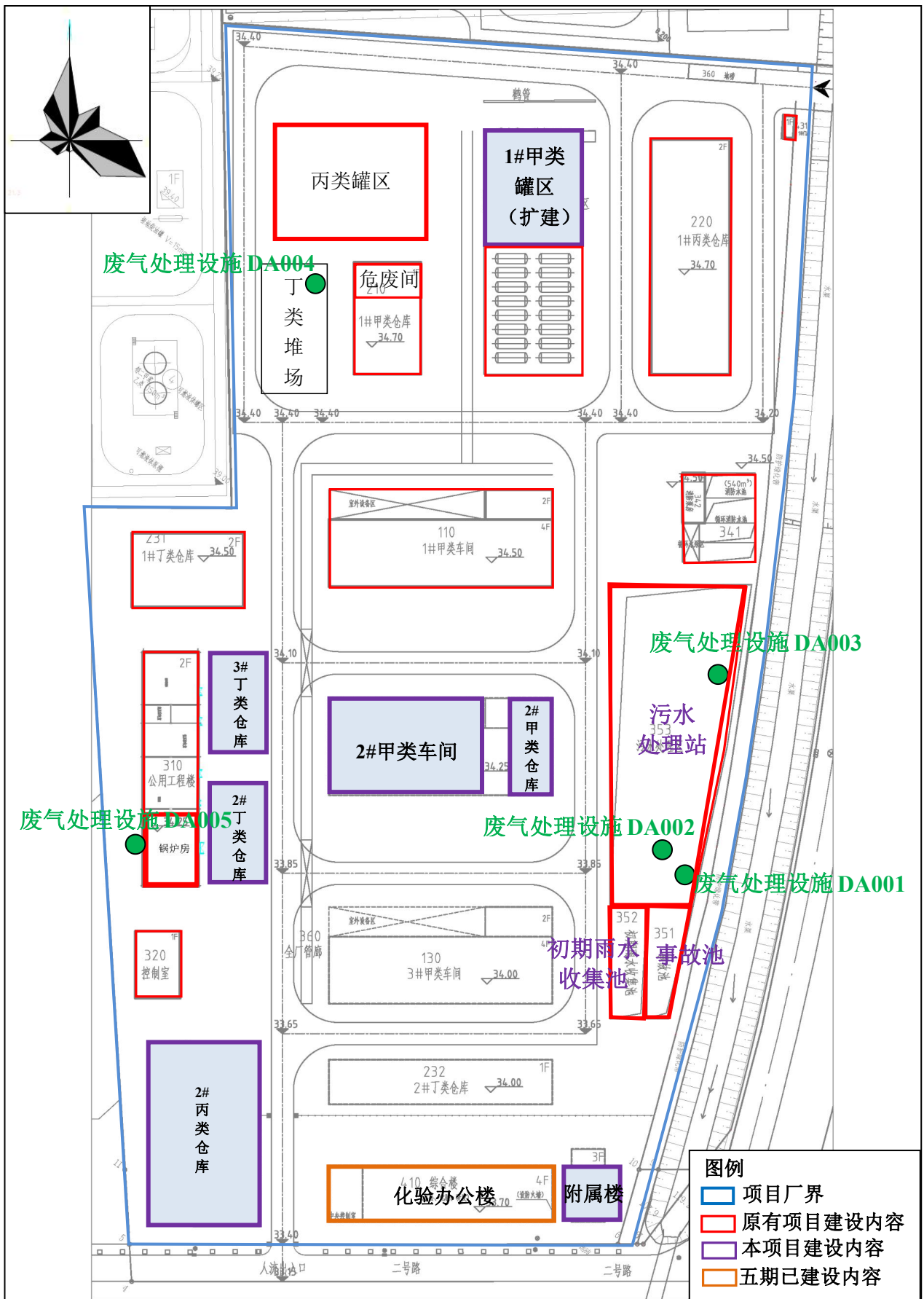
附图 5 项目厂区环保设施分布图
