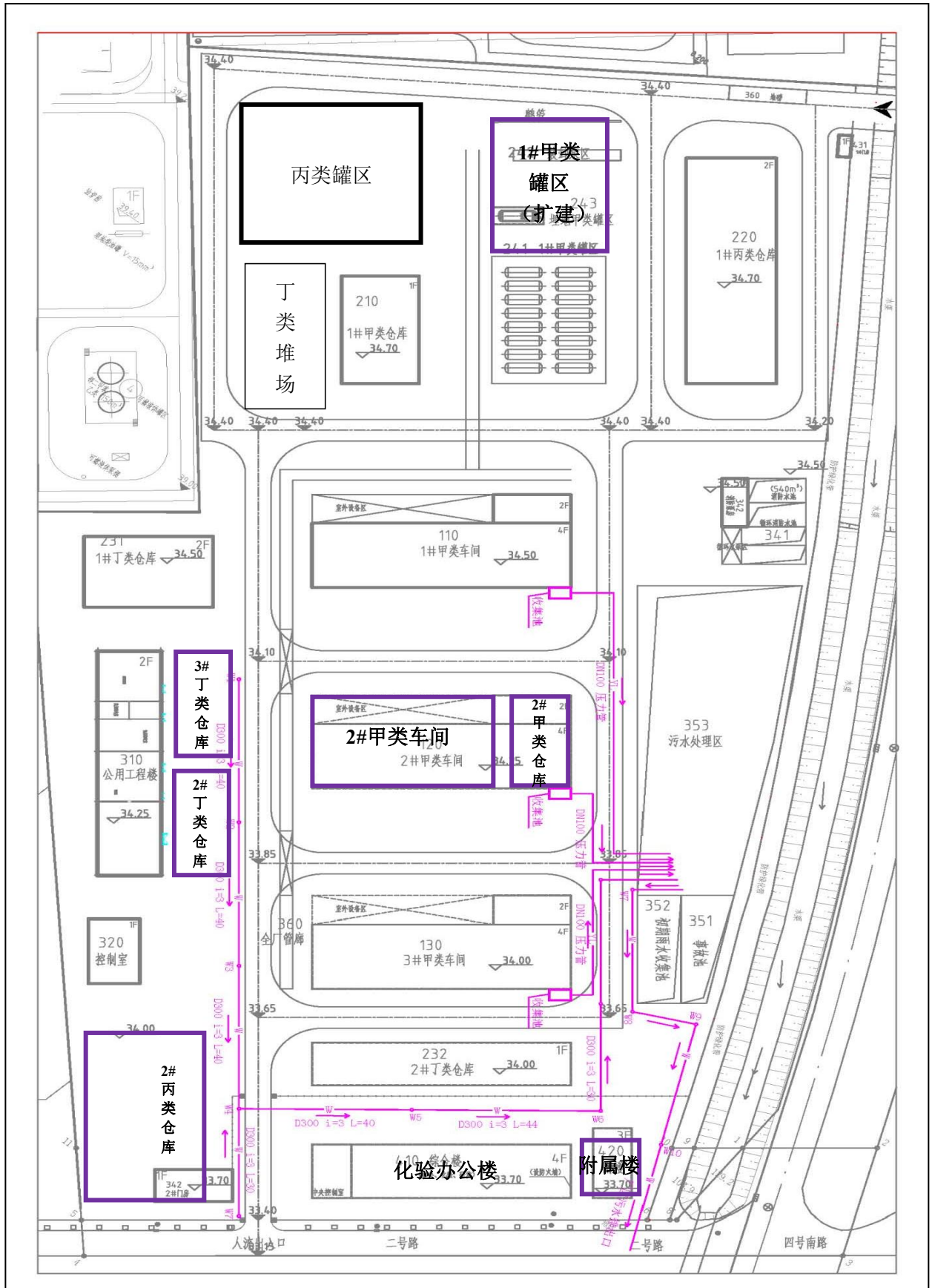
附图 7 项目厂区污水管道布置图
