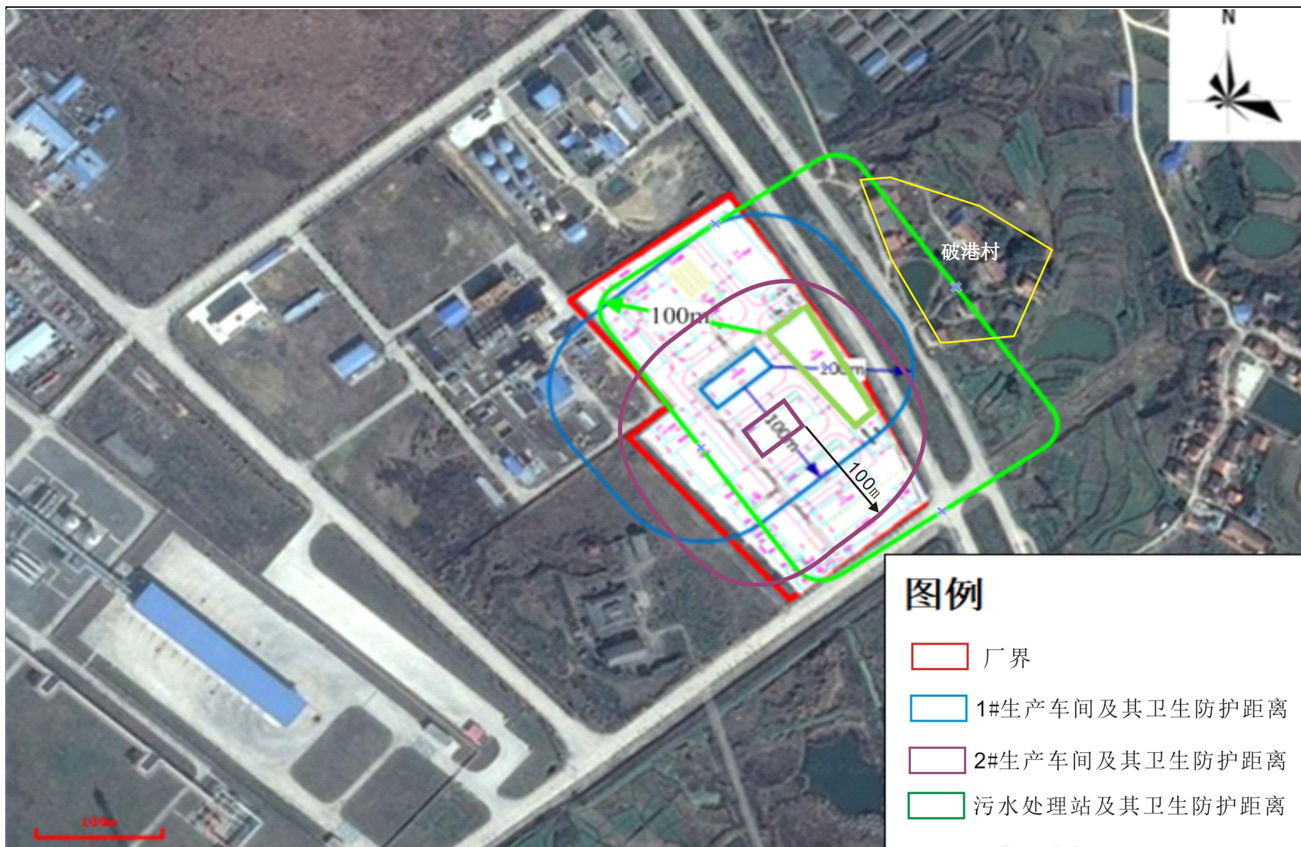
附图 11 卫生防护距离包络线图
