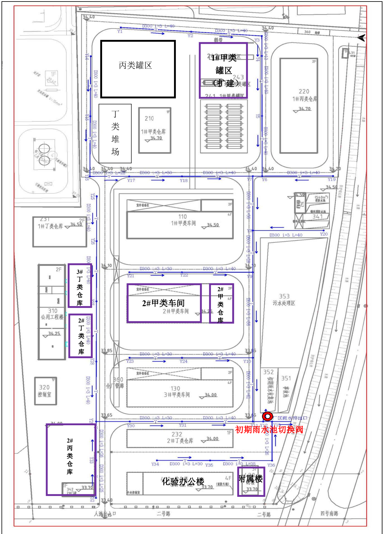
附图 8 项目厂区雨水管道布置图
