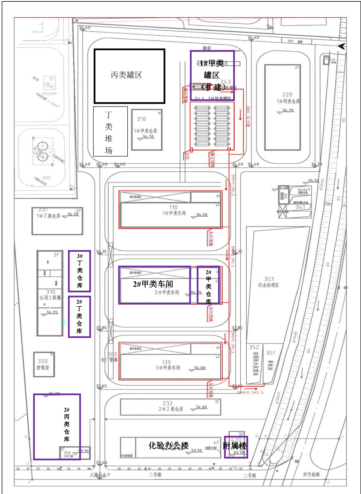
附图 9 项目厂区事故管道布置图
