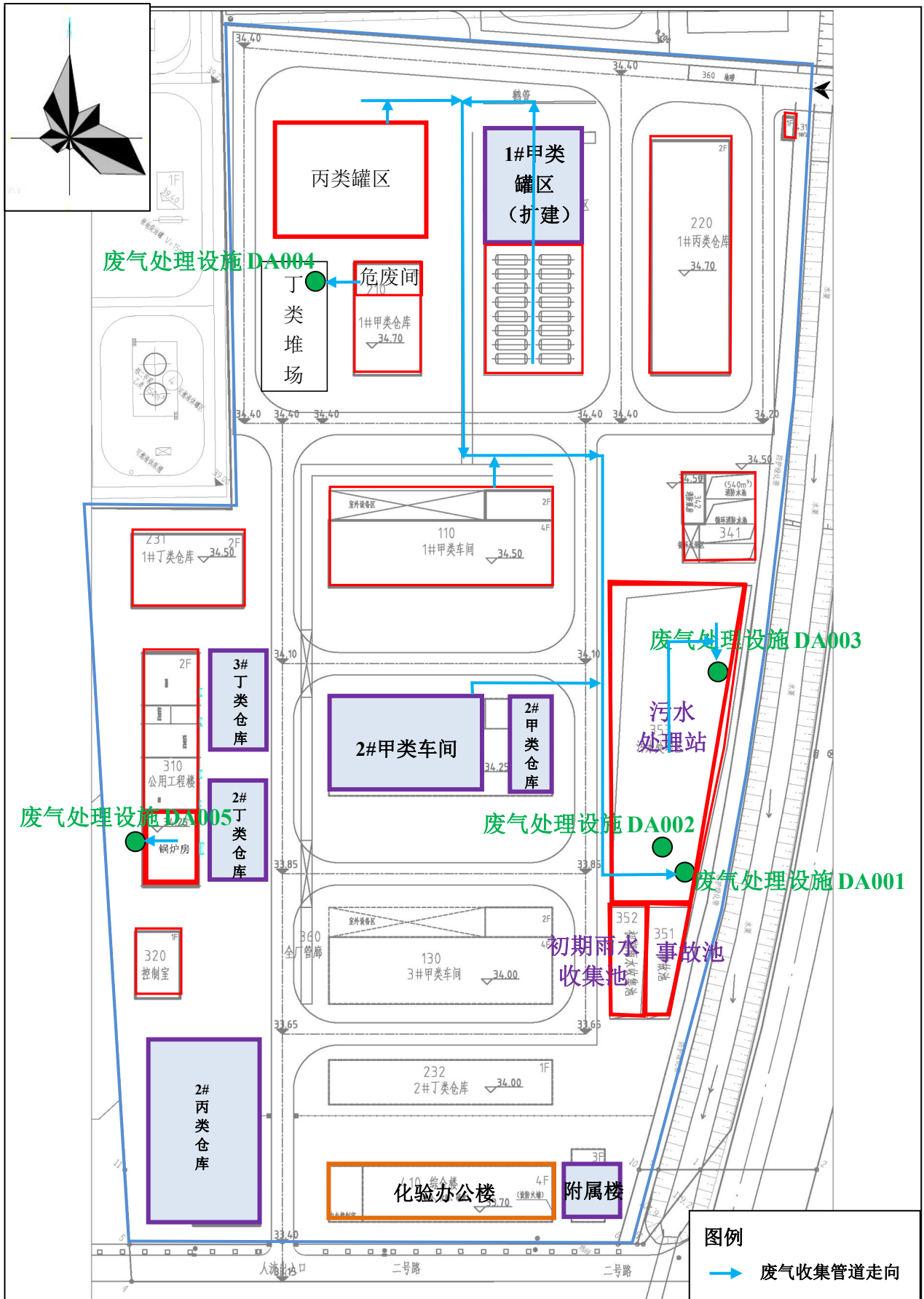
附图 6 项目废气收集图
